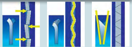
разведенные зубья волнообразные зубья заточенные зубья
